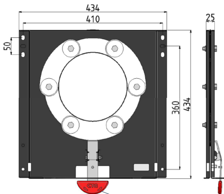
Leva di sgancio Release lever
